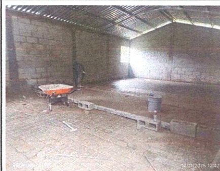
Foto 6: Fundición de piso
